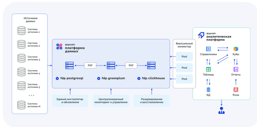
Сборка Clickhouse
